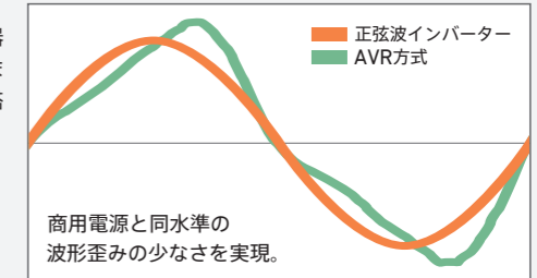
正弦波インバーター搭載発電機の出力波形イメージ
