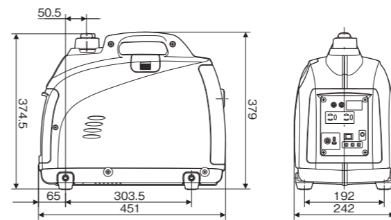
外観寸法図
